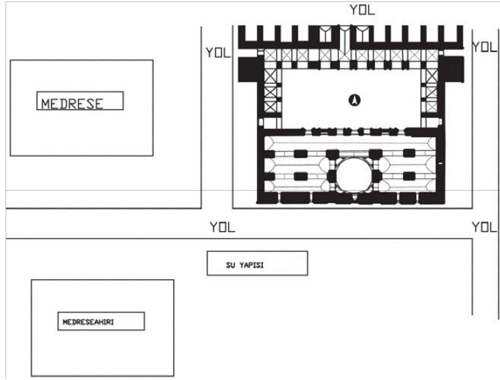
Çizim 2: Mardin Ulu Cami Külliyesi-Caminin Muhtemel İlk Vaziyet Planı (A. Gabriel'den işlenerek)
